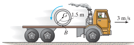
Prob. 16-90
