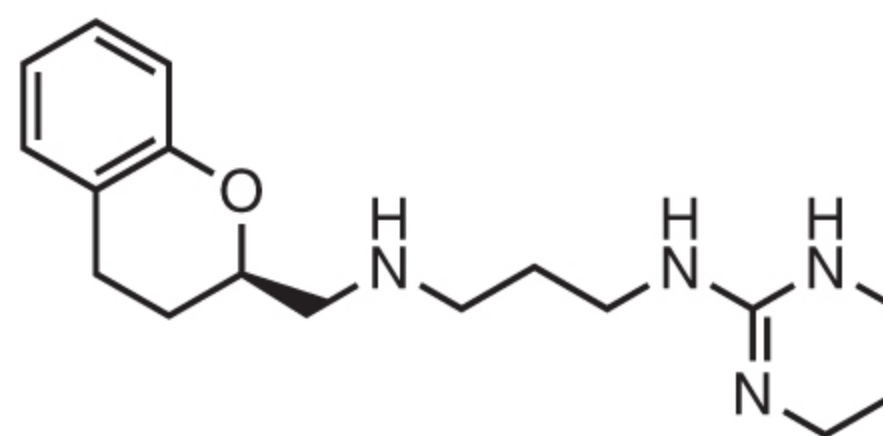
Alniditan
