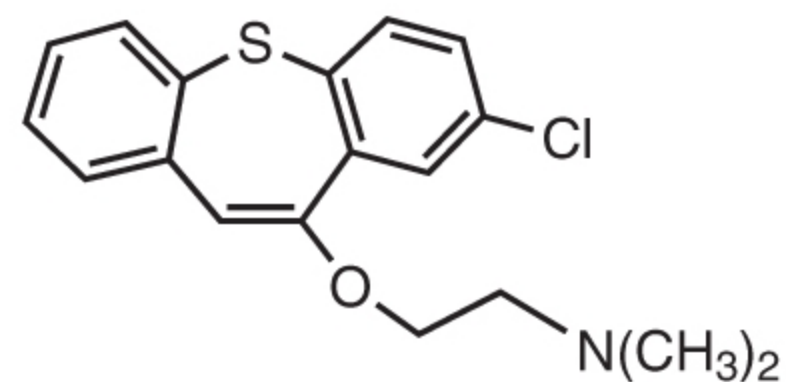
Zotepine
