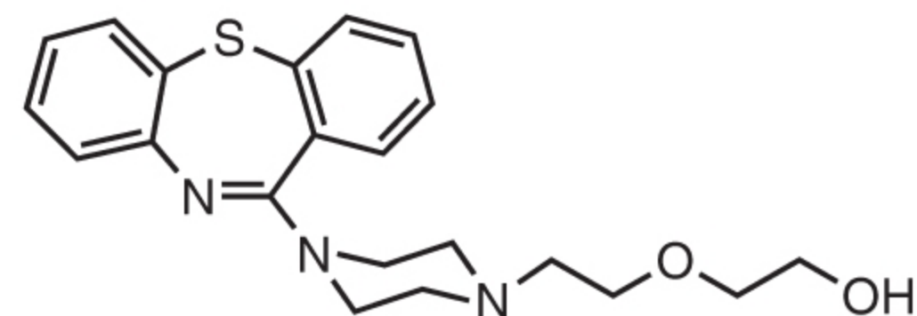
Quetiapine
