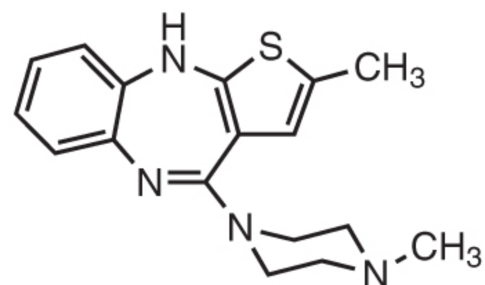
Olanzapine
