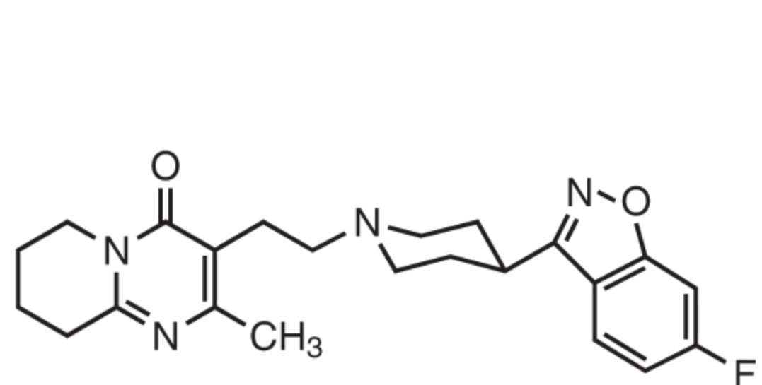
Risperidone
