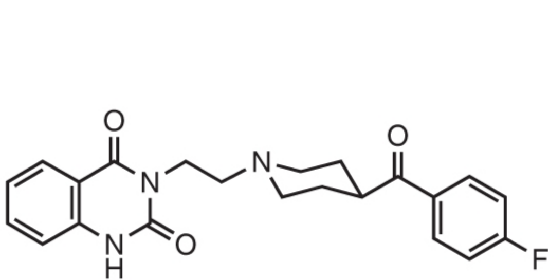
Ketanserin
