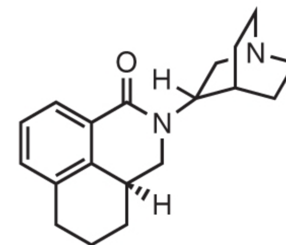
Palonosetron
