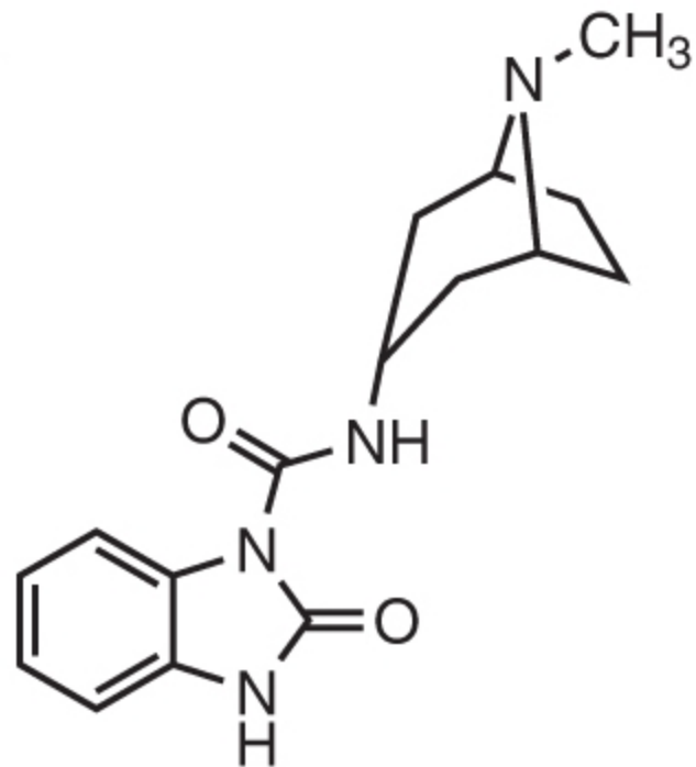
Itasetron
