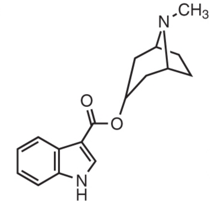
Tropisetron
