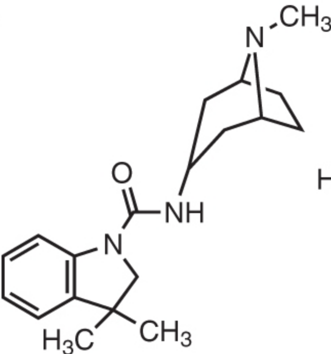
Ricasetron
