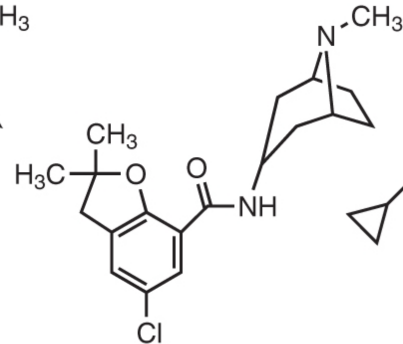
Zatosetron
