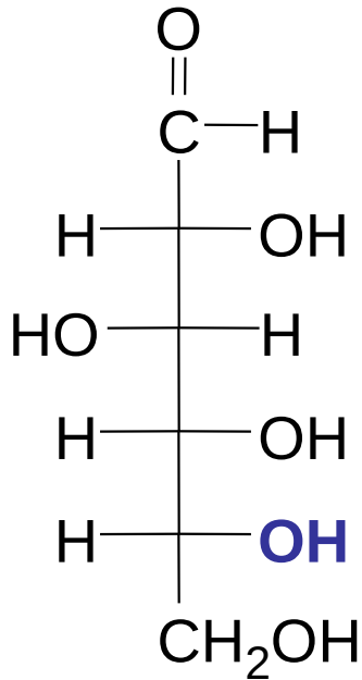
D -glucose
