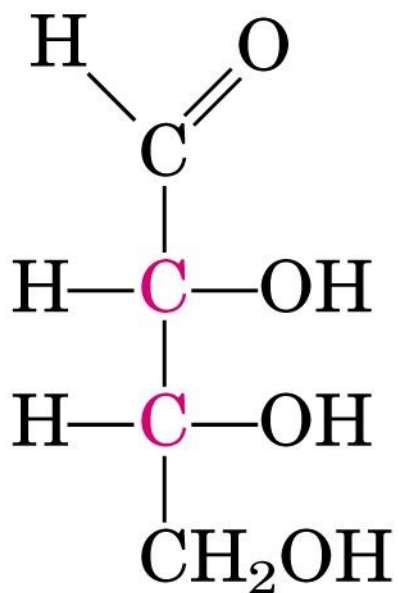
D-Erythrose
