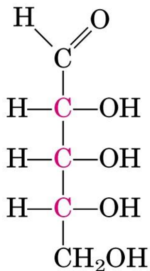
D-Ribose
