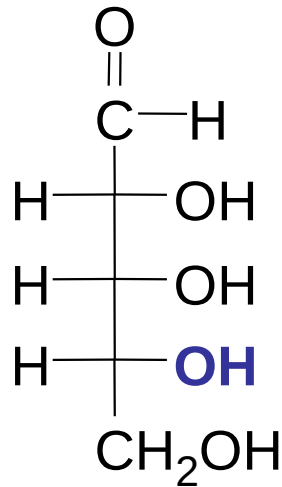
D -ribose
