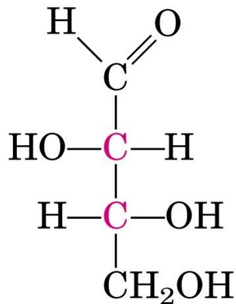
D-Threose
