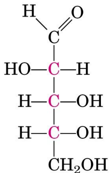
D-Arabinose
