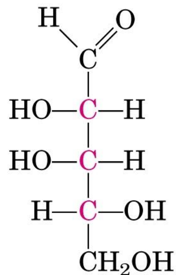
D-Lyxose
