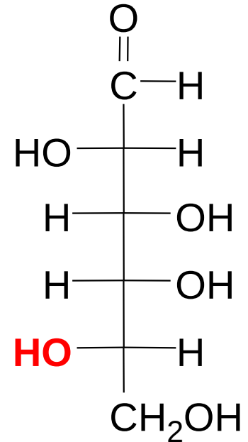
L -galactose
