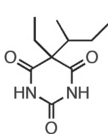
Butabarbital
