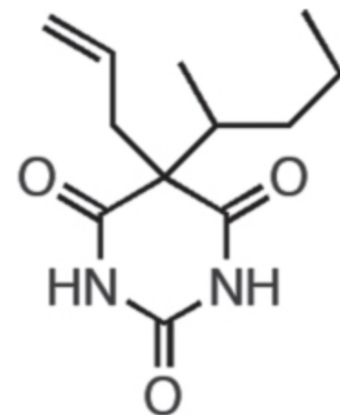
Secobarbital
