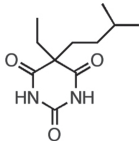
Amobarbital
