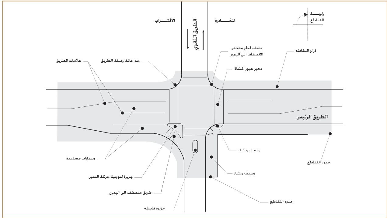
شكل 19: عناصر تخطيط وتصميم التقاطعات السطحية
