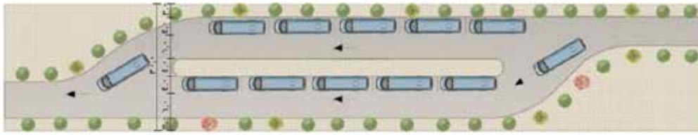
شكل 35: أنماط مختلفة من ساحات وقوف الحافلات (بالمتر)
