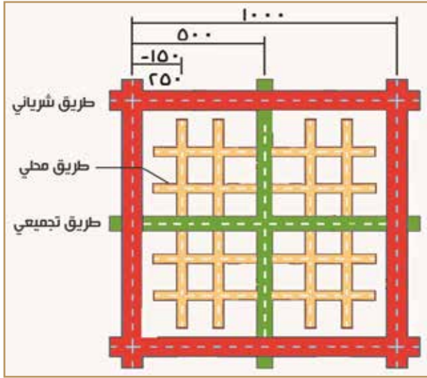
ويبين الشكل 45 نموذجاً للتباعد المثالي للتقاطعات في شبكة مفترضة. شكل 45: نموذج يبين التباعد بين التقاطعات (بالمتر)
