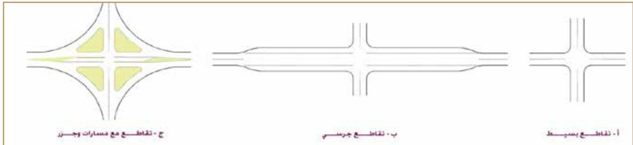
شكل 17: نماذج لأنواع مختلفة من التقاطعات ذات الأذرع الأربعة للطرق المتقاطعة على زاوية قائمة
