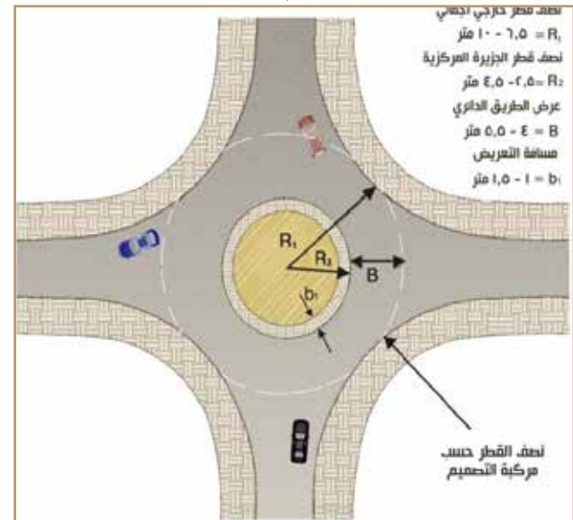
شكل 28: تصميم الدوار الصغير
