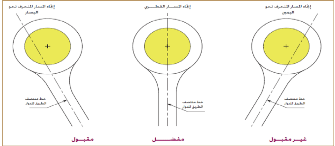
شكل 27: التخطيط القطري لساكنات الطرق المقترية من مدخل الدوار
