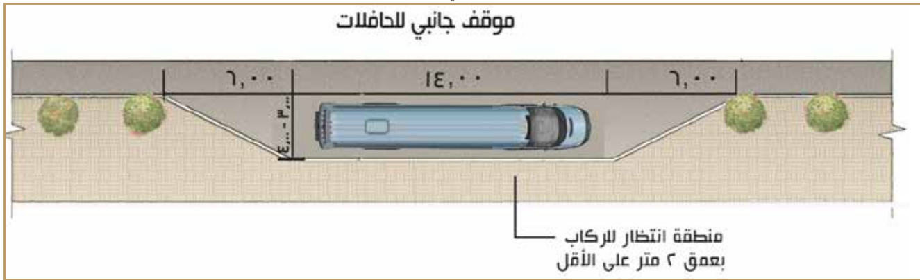
شكل 34: نموذج لموقف جانبي للحافلات مواز لمسارب الحركة (بالمتر)
