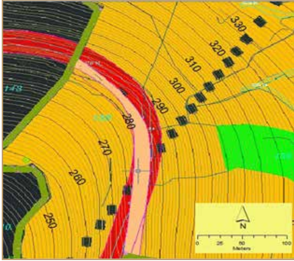
شكل 41: اختيار موقع الطريق مع الأخذ بالاعتبار طبوغرافيا المنطقة
