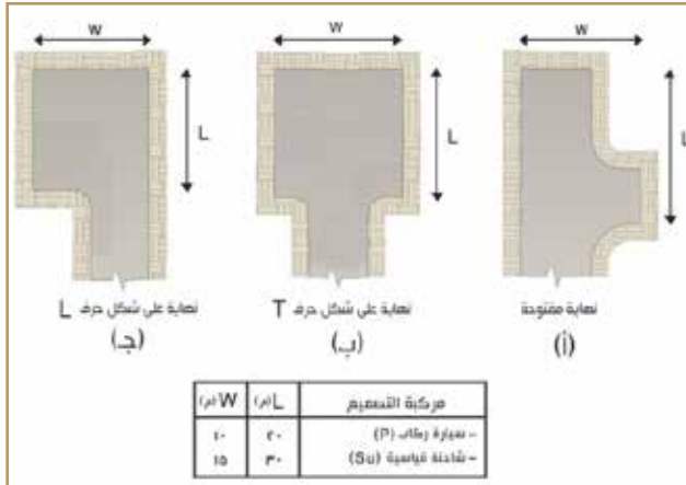
شكل 32: نماذج لطريق غير نافذة مع نهاية مستطيلة
