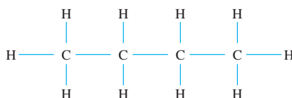
Butane
