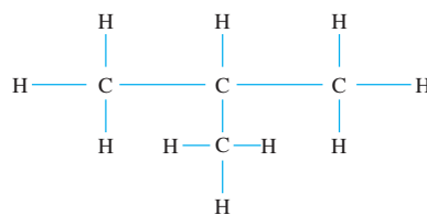
Isobutane
