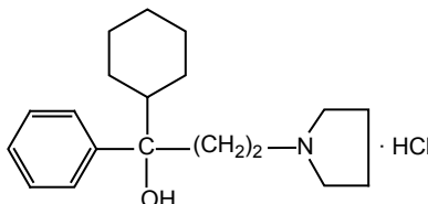
1-Cyclohexyl-1-phenyl-3-pyrrolidin-1-yl-1-propanol HCl
