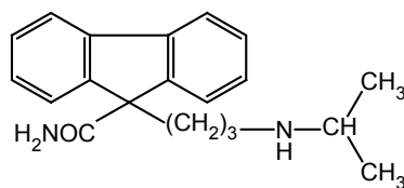
Indecainide
