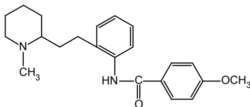
Encainide
