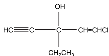
Ethychlorvynol
