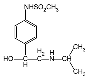
talol
