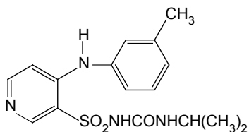
Toresemide
