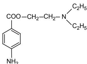
Procaine
