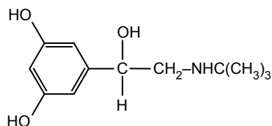
j. Terbutaline
