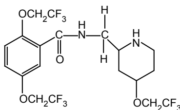
Flecainide
