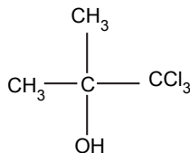
Chlorbutanol
