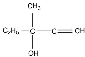
Methyl pentynol
