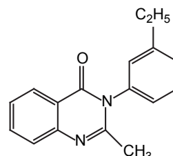
Ethinazone
