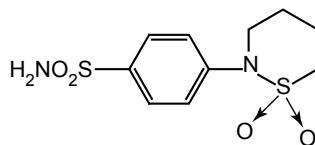
Sulthiame
