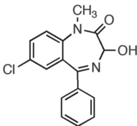
Temazepam
