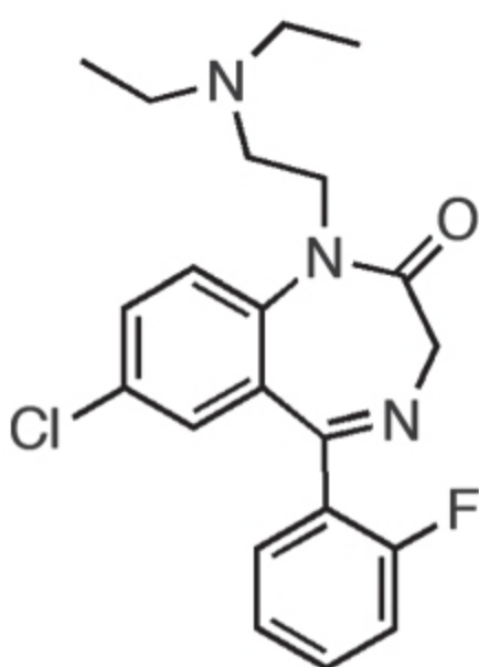
Flurazepam
