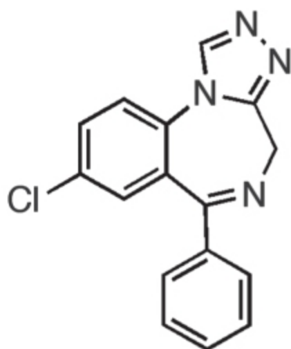
Estazolam
