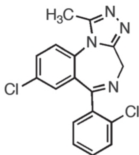
Triazolam
