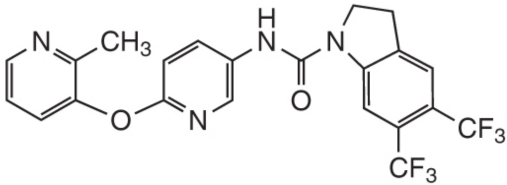
SB-243213
