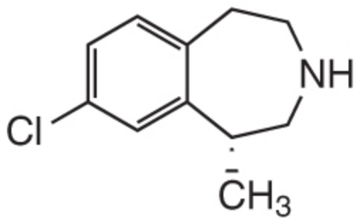
Lorcaserin
